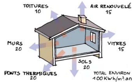
les pertes de chaleur d'une maison individuelle isolée RT2005
